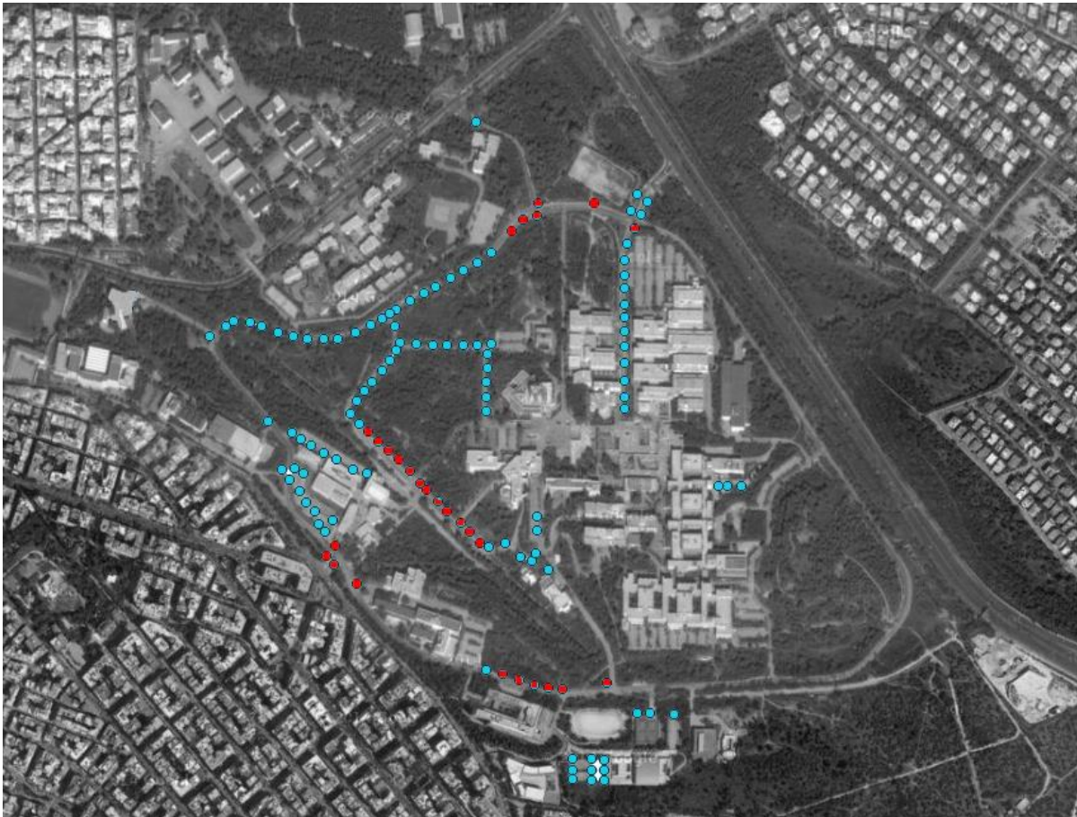
Εικόνα 2 HPS-STR-1 (2/3). Τα φωτιστικά απεικονίζονται με κόκκινο χρώμα. Φωτιστικά οδών.
