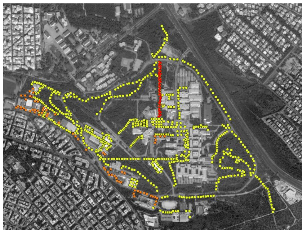
Εικόνα 8 Φωτιστικά οδικού τύπου που ανήκουν στην CFL-PED-2 (2/2) (κόκκινο χρώμα)
